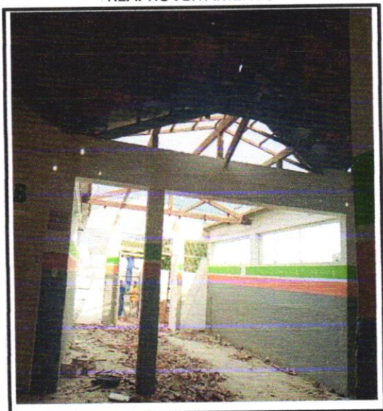
FOTO - 01 REMOÇÃO DE TRAMA DE MADEIRA PARA COBERTURA, DE FORMAMANUAL, SEM REAPROVEITAMENTO
