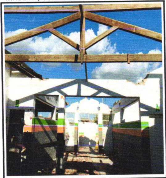
FOTO - 03 : REMOÇÃO DE TESOURAS DE MADEIRA, COM VÃO MAIOR OU IGUAL A 8M,
